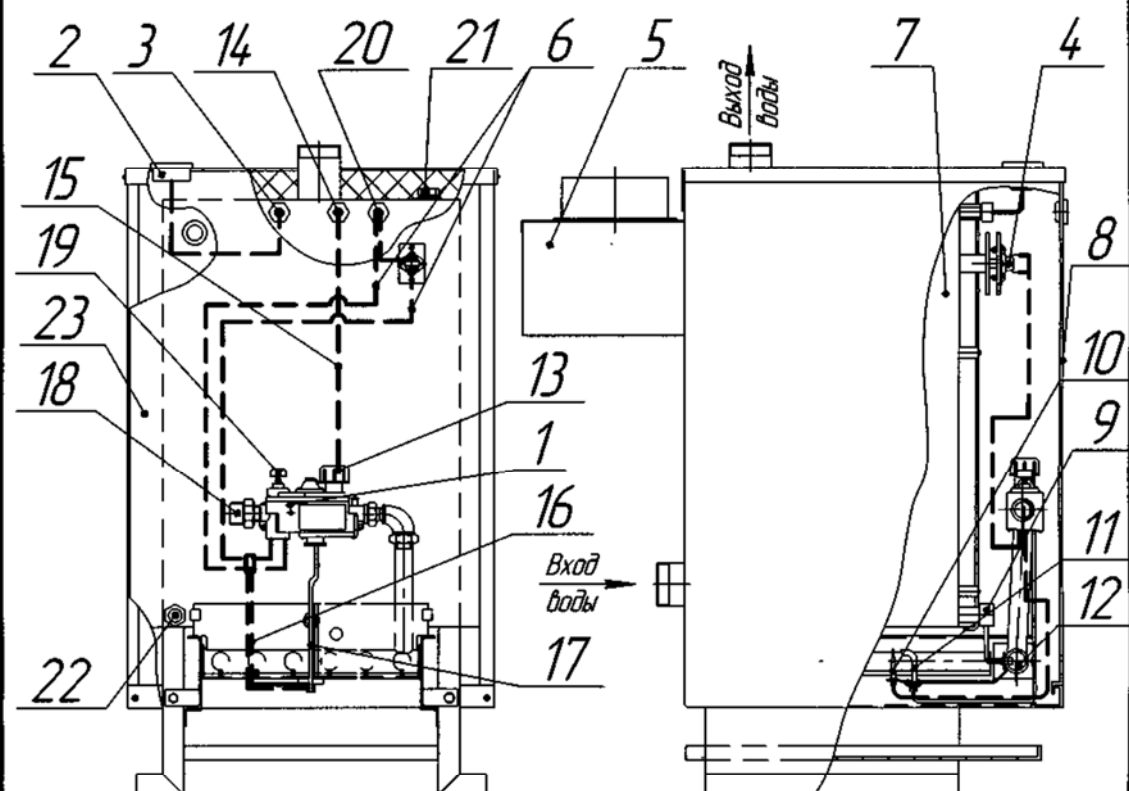
Рис. 2. Конструкция котла.
